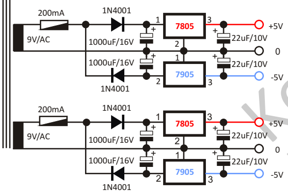
SIMETRIČNO NAPAJANJE ZA DIGITALNI VOLTMETAR
